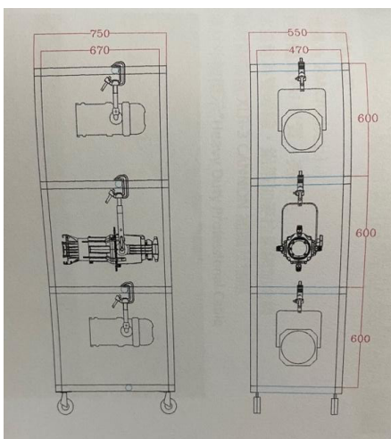
活動式側燈燈光架
