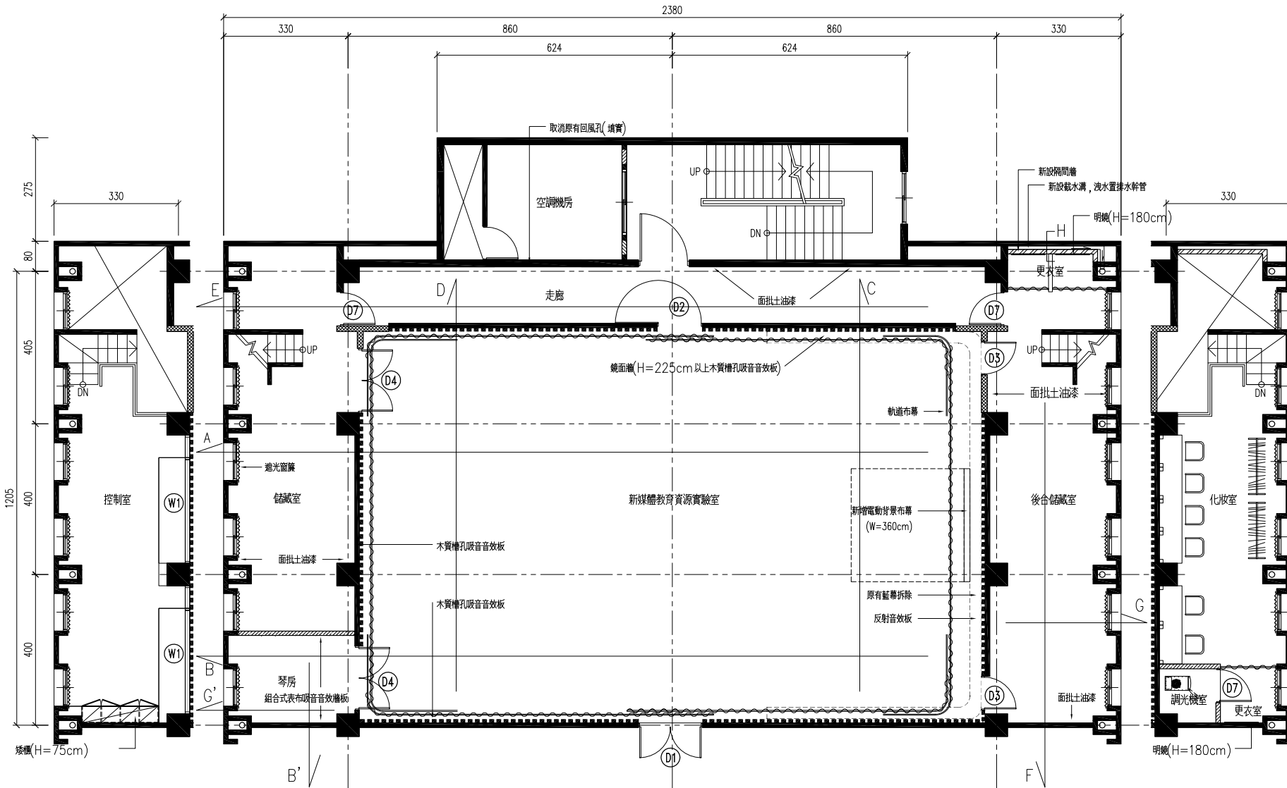
圖書館校區綜合大樓十樓 教育資源實驗室(夾層)平面配置圖 S:1/100
